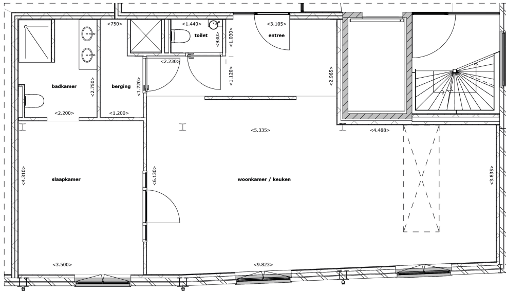
Plattegrond verdieping 03 1:50
